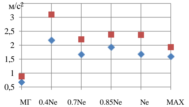
Рисунок 1. Зависимость интенсивности составляющей 1/3 f_{z1} от режима работы двигателя при двух вариантах бокового зазора: \blacklozenge - 0.30 мм, \blacksquare - 0.43 мм
