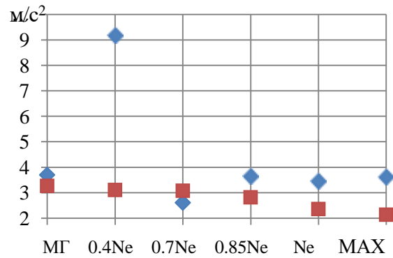
Рисунок 2. Зависимость интенсивности составляющей 2/3 f_{z1} от режима работы двигателя при двух вариантах бокового зазора: \blacklozenge - 0.30 мм, \blacksquare - 0.43 мм
