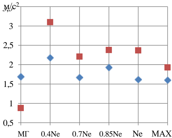
Рисунок 4. Зависимость интенсивности составляющей f_{изн} от режима работы двигателя при двух вариантах бокового зазора: \blacklozenge – 0.30 мм, \blacksquare – 0.43 мм
